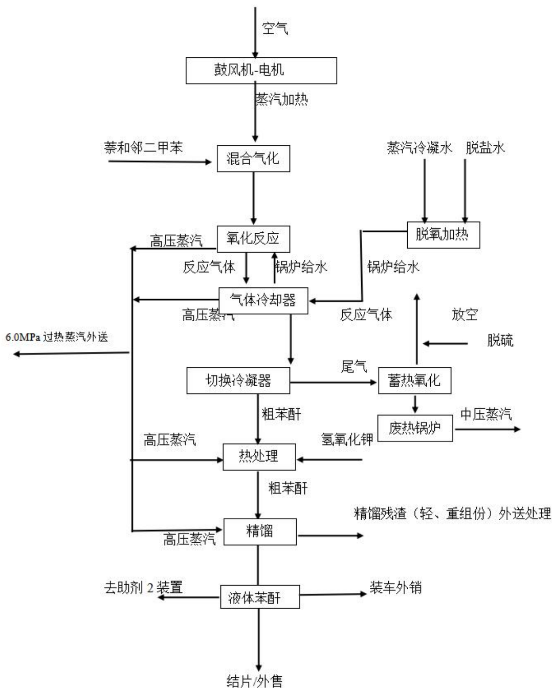
图 3-4 苯酐生产工艺流程图
