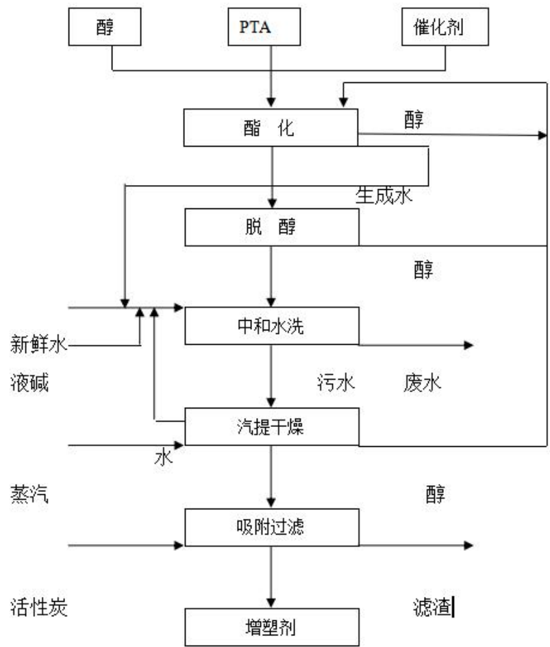
图 3.1 环保增塑剂生产流程图
